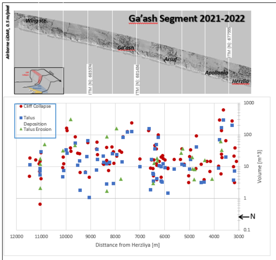
איור 9. סיכום פעילות המצוק לאורך מקטע געש 2021 - 2022 מוצגת לפי המרחק ממרינת הרצליה. אדום: קריסת מצוק, כחול: השקעת טאלוס, ירוק: סחיפת טאלוס על ידי הגלים (מוצג בצורה סכמתית באיור המוקטן). קואורדינטות צפון ברשת ישראל החדשה באפור.
