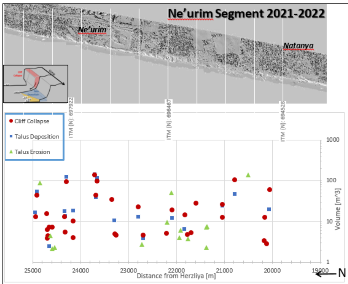
איור 6. סיכום פעילות המצוק לאורך מקטע נעורים 2021 - 2022 מוצגת לפי המרחק ממרינת הרצליה. אדום: קריסת מצוק, כחול: השקעת טאלוס, ירוק: סחיפת טאלוס על ידי הגלים (מוצג בצורה סכמתית באיור המוקטן). קואורדינטות צפון ברשת ישראל החדשה באפור.
