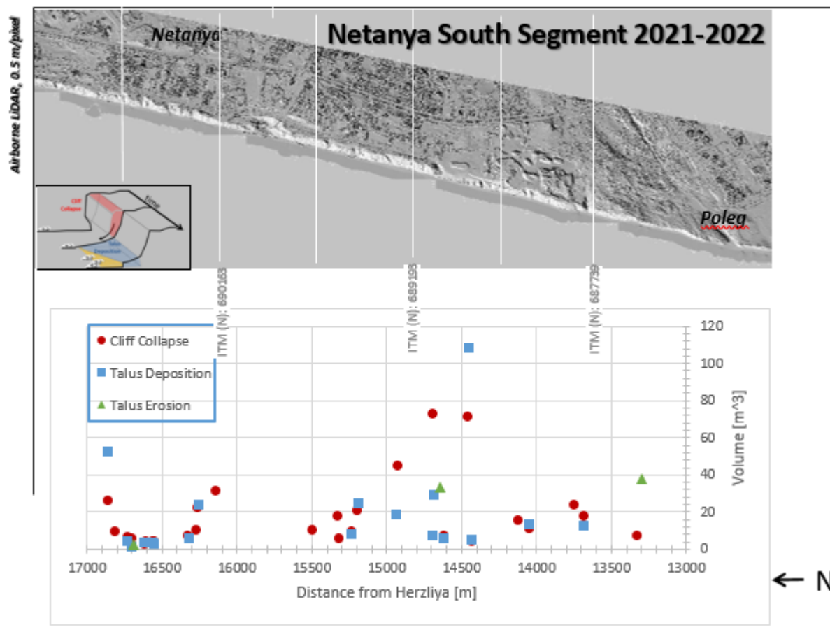
איור 8. סיכום פעילות המצוק לאורך מקטע נתניה דרום 2021 - 2022 מוצגת לפי המרחק ממרינת הרצליה. אדום: קריסת מצוק, כחול: השקעת טאלוס, ירוק: סחיפת טאלוס על ידי הגלים (מוצג בצורה סכמתית באיור המוקטן). קואורדינטות צפון ברשת ישראל החדשה באפור.
