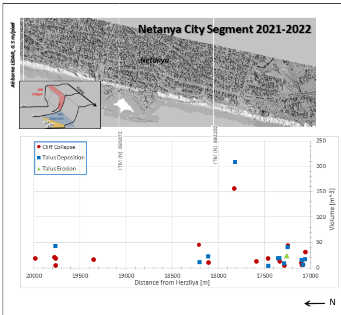
איור 7. סיכום פעילות המצוק לאורך מקטע נתניה העיר 2021 - 2022 מוצגת לפי המרחק ממרינת הרצליה. אדום: קריסת מצוק, כחול: השקעת טאלוס, ירוק: סחיפת טאלוס על ידי הגלים (מוצג בצורה סכמטית באיור המוקטן). קואורדינטות צפון ברשת ישראל החדשה באפור.
