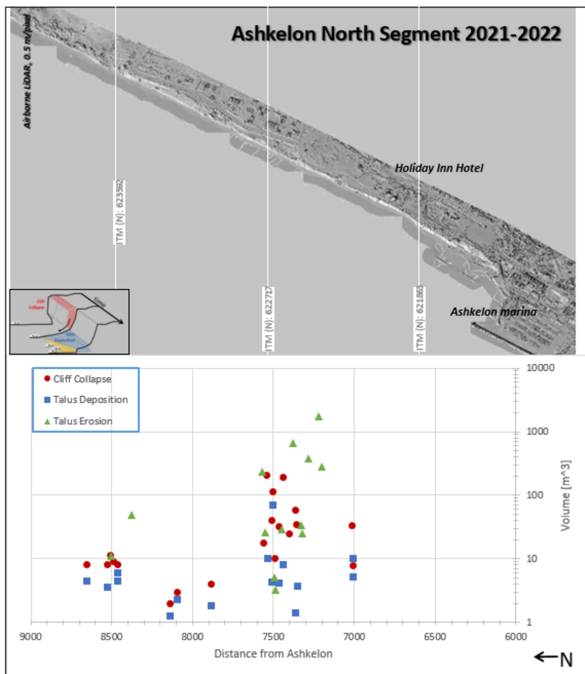
איור 10. סיכום פעילות המצוק לאורך מקטע אשקלון צפון 2021 - 2022 מוצגת לפי המרחק מתחנת הכוח. אדום: קריסת מצוק, כחול: השקעת טאלוס, ירוק: סחיפת טאלוס על ידי הגלים (מוצג בצורה סכמתית באיור המוקטן). קואורדינטות צפון ברשת ישראל החדשה באפור.
