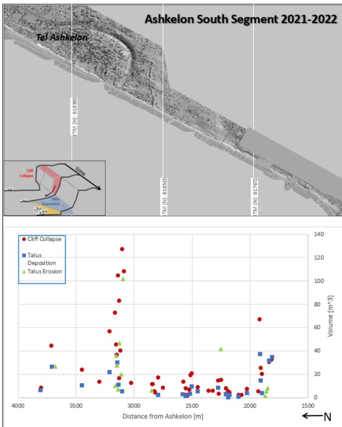
איור 11. סיכום פעילות המצוק לאורך מקטע אשקלון דרום 2021 - 2022 מוצגת לפי המרחק מתחנת הכוח. אדום: קריסת מצוק, כחול: השקעת טאלוס, ירוק: סחיפת טאלוס על ידי הגלים (מוצג בצורה סכמתית באיור המוקטן). קואורדינטות צפון ברשת ישראל החדשה באפור.
