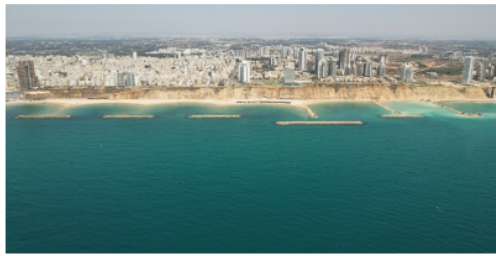
פרויקט שוברי הגלים בנתניה | צילום: החברה הממשלתית להגנות מצוקי חוף הים התיכון
